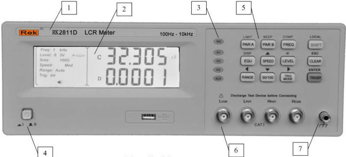
图2-1 前面板
